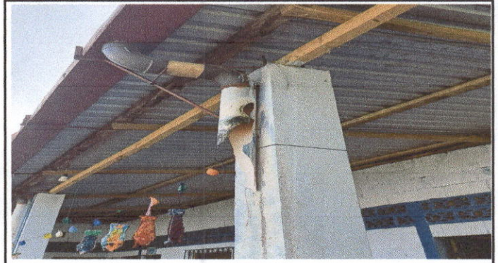
sustitución de la bajada de agua pluvial, sustitución de soporte de madera por metal, mantenimiento del canal de metal, Modulo 3 corredor
